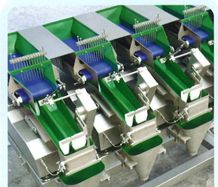
Peseuses linéaires, exécutions spécifiques pour produits collants, facilité de nettoyage
