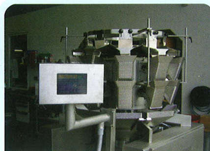
Peseuses associatives: - pour environnements difficiles - mini-doses à partir de 1 gr.
