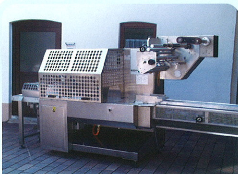
Ensacheuses horizontales cadences de 45 à 450 sachets/minute avec ou sans barquette, longueur variable des produits. Execution inox possible Films : Polyéthylène ou complexe
