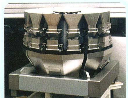
Peseuses associatives de 10 à 24 têtes de construction acier inoxydable. Station de transfert vers thermoformeuses. Multi-produits - mélanges
